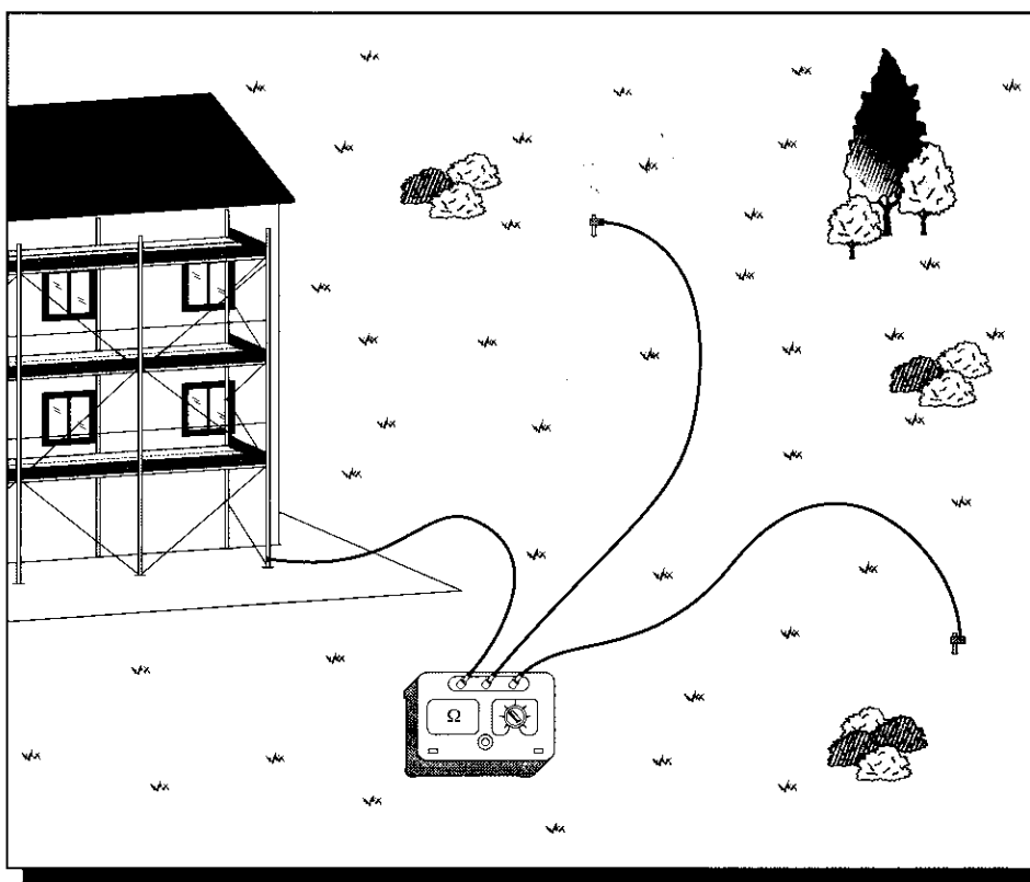
Fig. 3 - Misura della resistenza di terra naturale del ponteggio.
