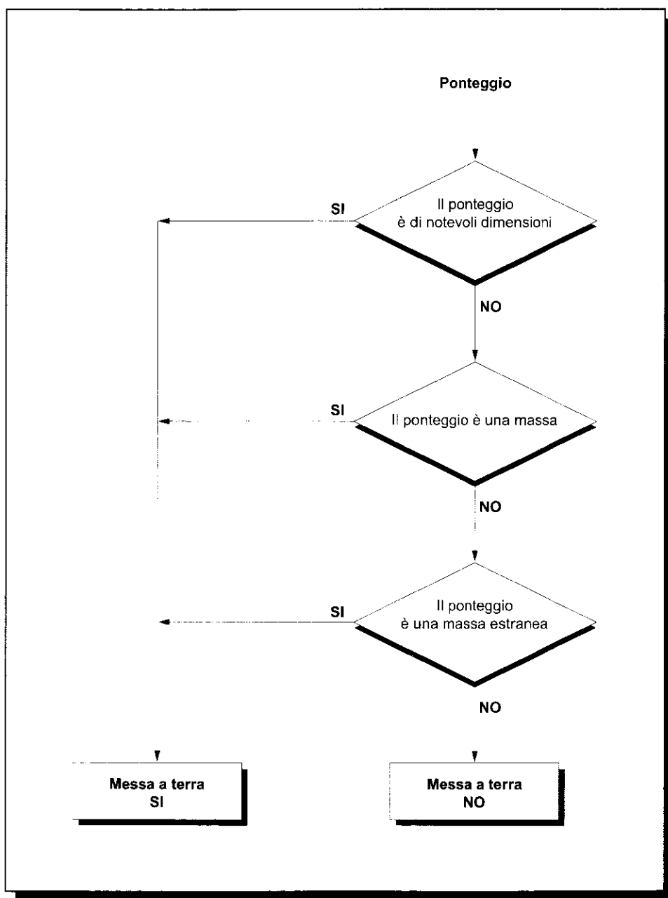
Fig. 4 - Il ponteggio va collegato a terra solo in casi particolari.
