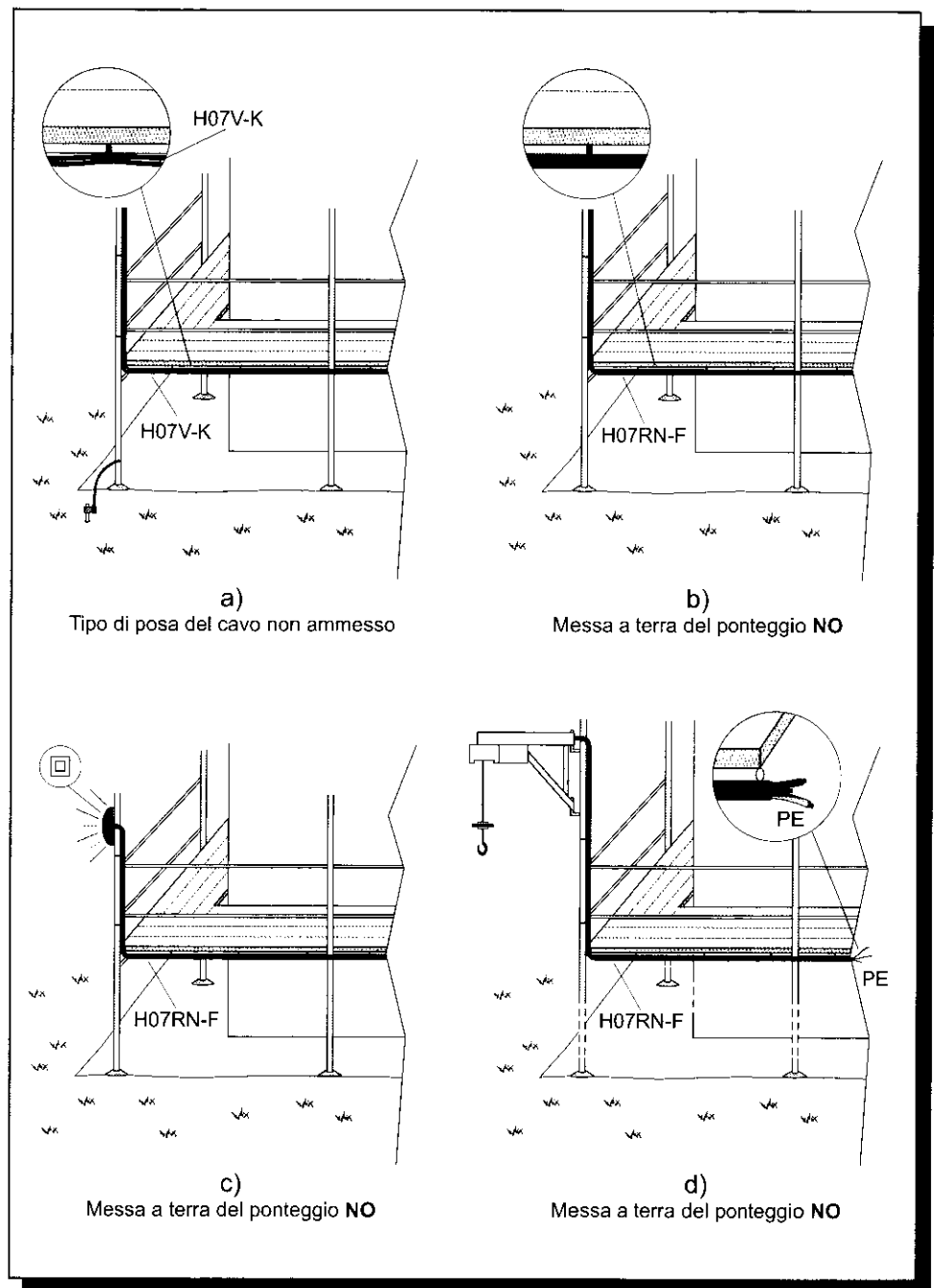
Fig. 1 - Messa a terra del ponteggio.
