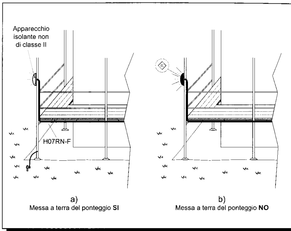
Fig. 2 - Messa a terra del ponteggio.
